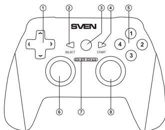
Рис. 1. Вид сверху
