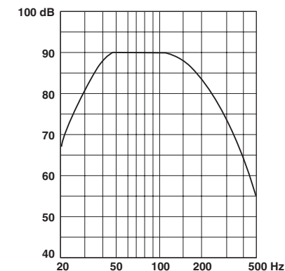
Diagram van de frequentiecarakteristieken*
