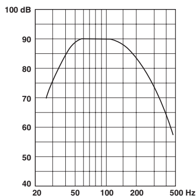
Diagram van de frequentiecarakteristieken*
