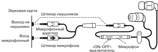
Рис. 1. Схема подключения
