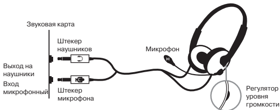
Рис. 1. Схема подключения
