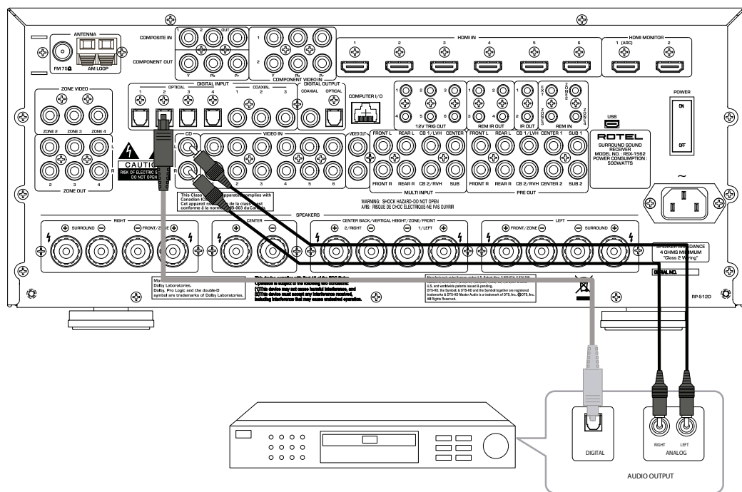
Рис. 8: Подключения CD-плеера
