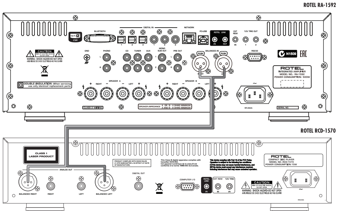
Figure 5: Balanced (XLR) Inputs Entrées symétriques (XLR) Anschlussdiagramm (symmetrische (XLR-) Eingänge) Entradas Balanceadas (XLR)
