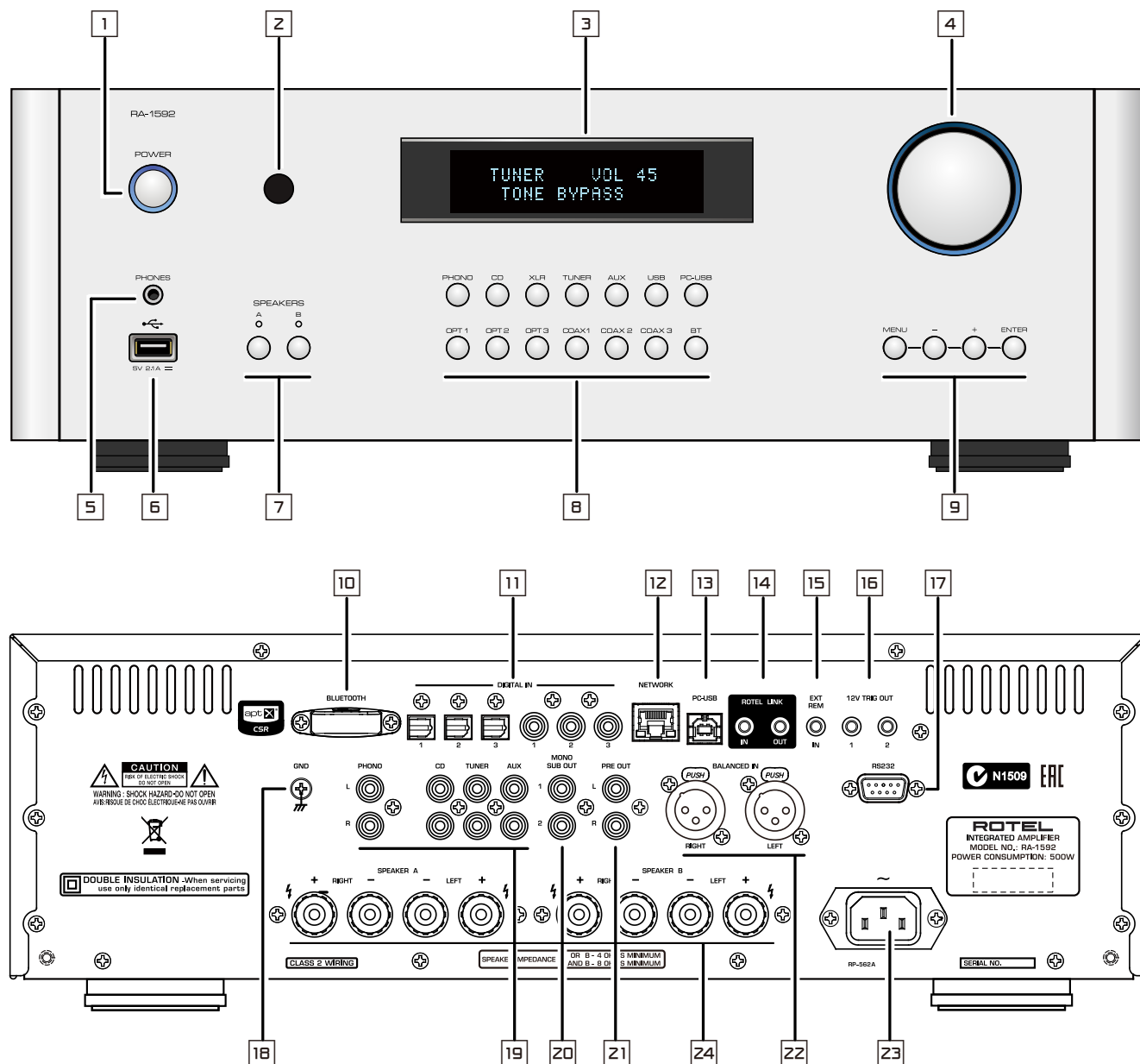
Figure 1: Controls and Connections Commandes et Branchements Bedienelemente und Anschlüsse Controles y Conexiones Bedieningselementen en aansluitingen ontrolli e connessioni e anslutningar Органы управления и разъемы
