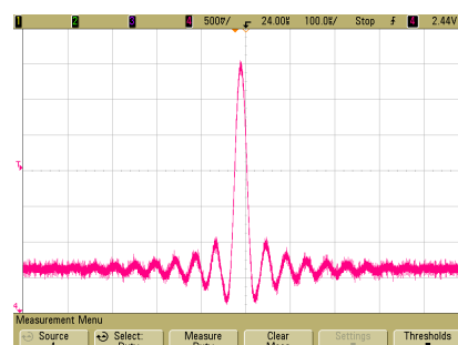
Импульсная характеристика цифрового фильтра FIR устройства CAS192D
