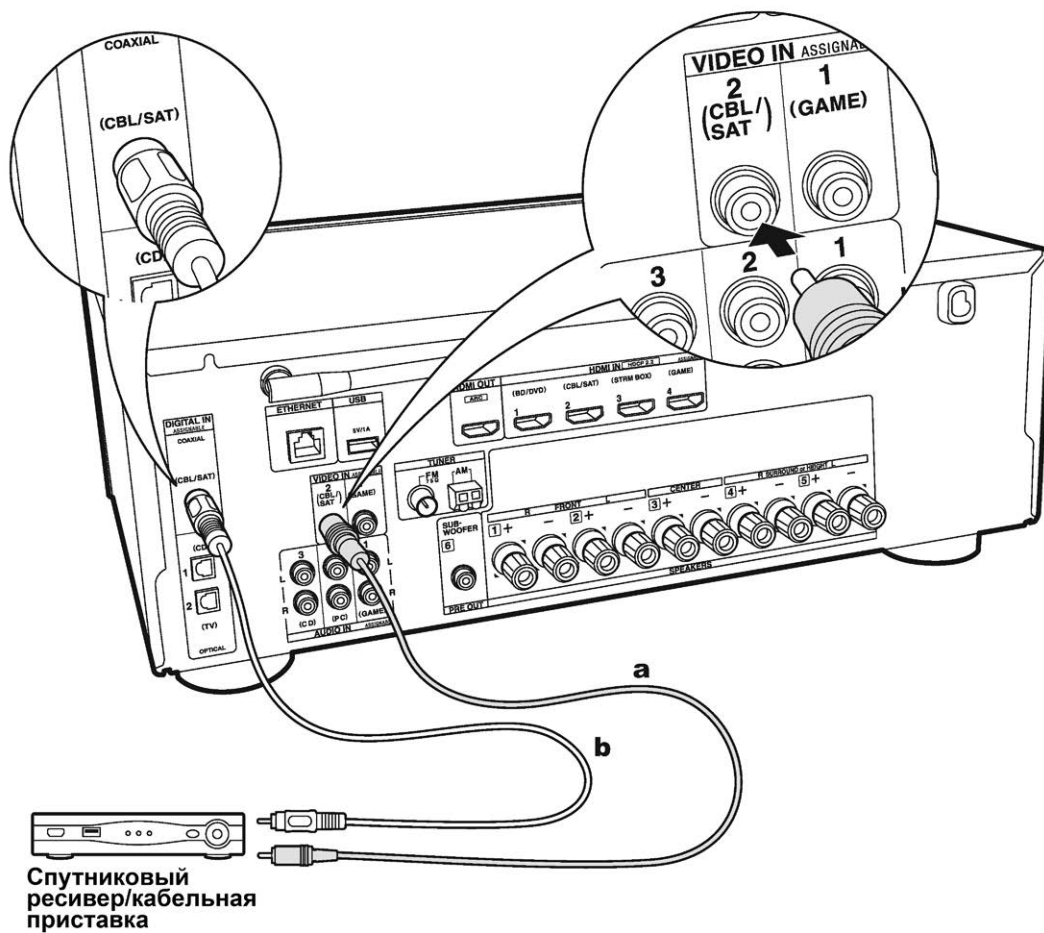
a аналоговый видео кабель, b цифровой коаксиальный кабель
