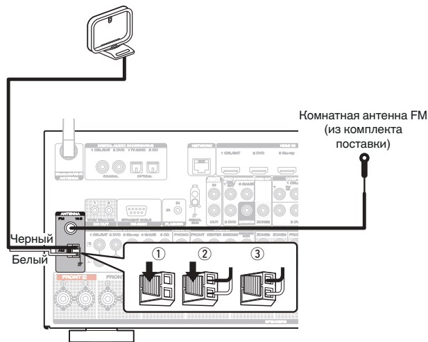
Рамочная AM-антенна (из комплекта поставки)
