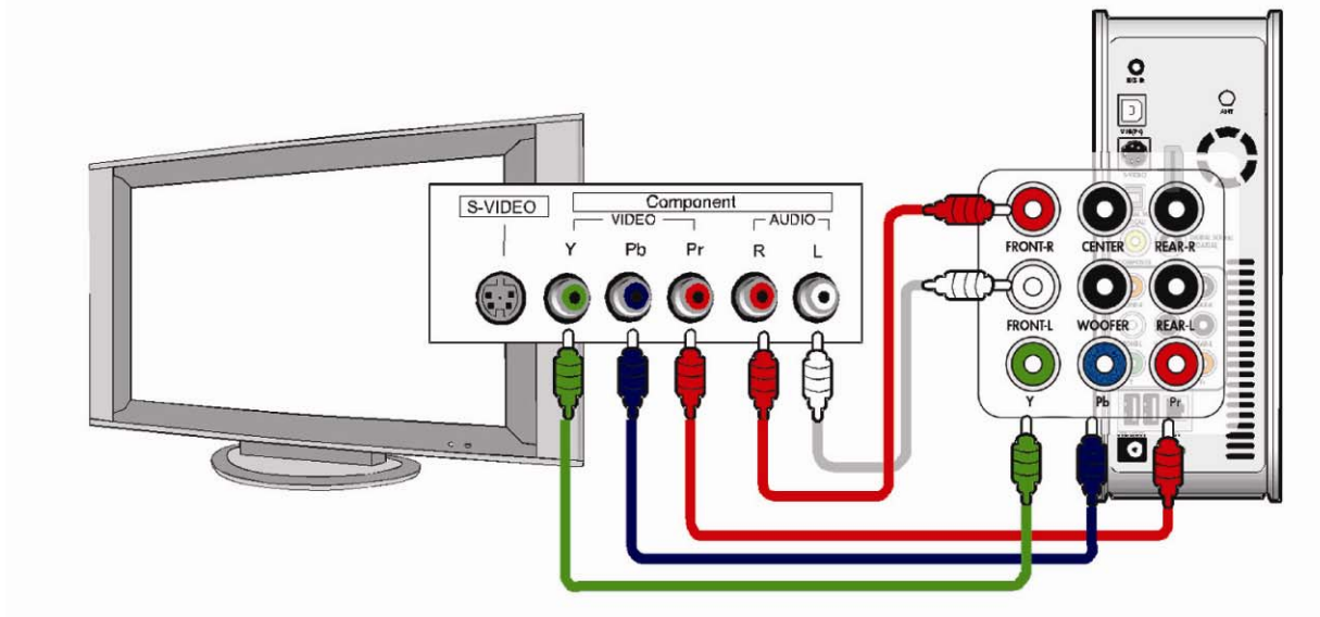
Соединение при помощи компонентного кабеля
