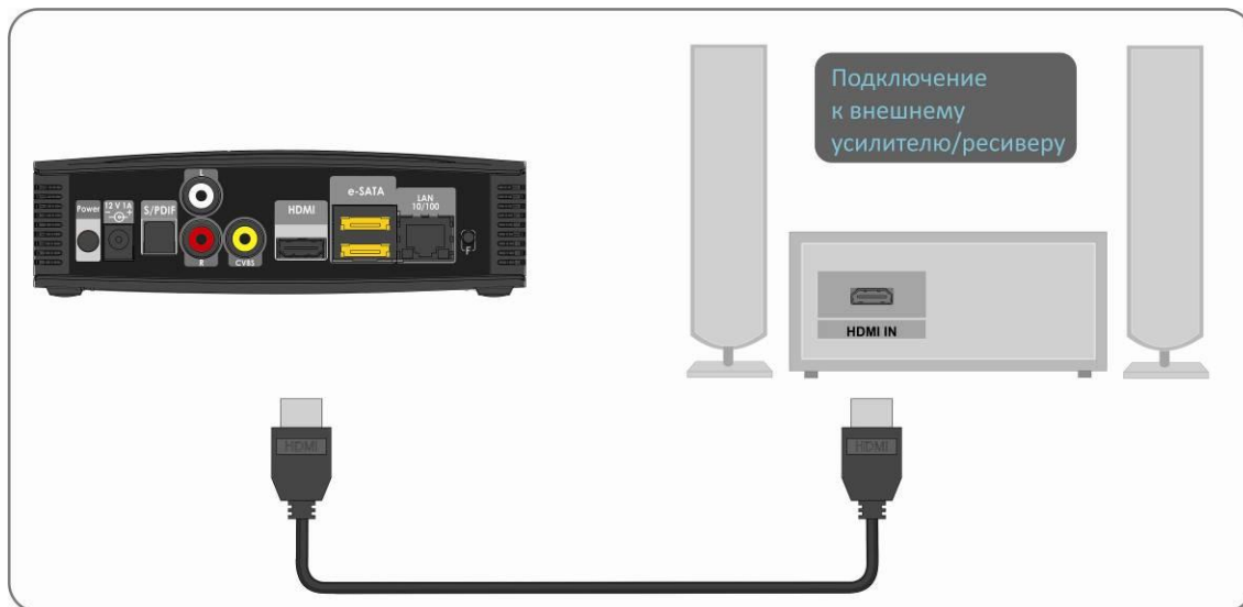
Рисунок 15 – Подключение STB NV-101 к акустической системе с разъемом HDMI
