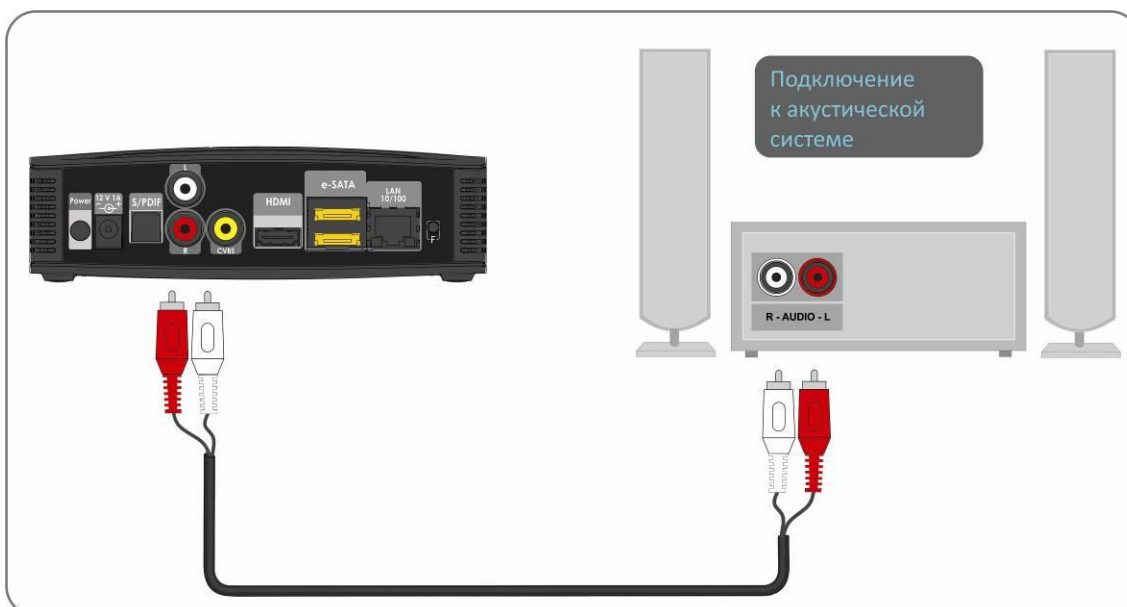
Рисунок 14 – Подключение к акустической системе с аналоговым аудиовходом RCA
