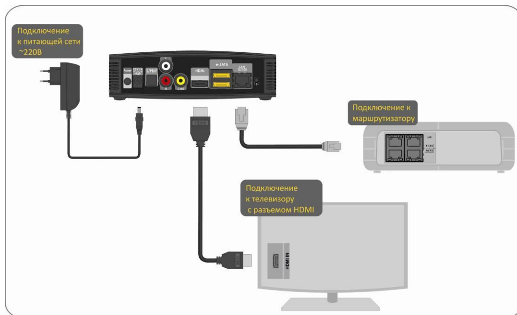
Рисунок 11 – Пример подключения STB NV-101
