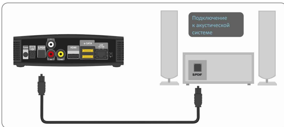
Рисунок 13 – Подключение к акустической системе с аудиовходом S/PDIF
