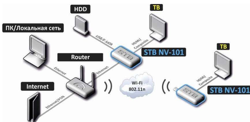
Рисунок 1 – Схема применения
