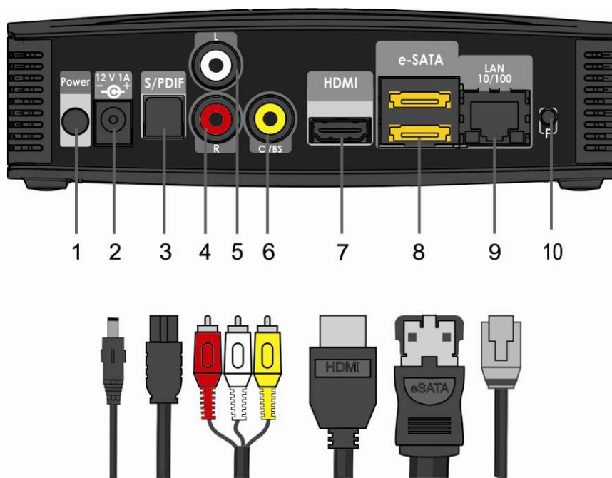
Рисунок 3 – Внешний вид задней панели STB NV-101
