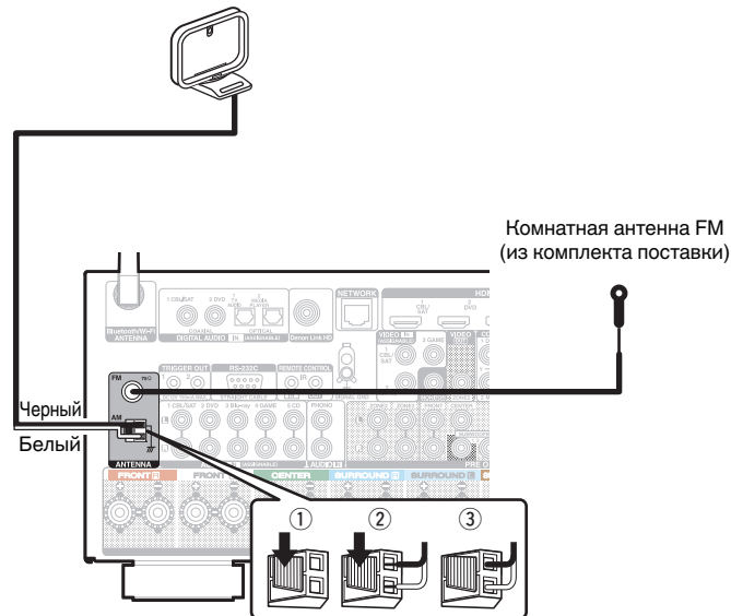
Рамочная AM-антенна (из комплекта поставки)
