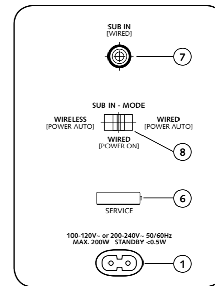
Subwoofer DM 900
