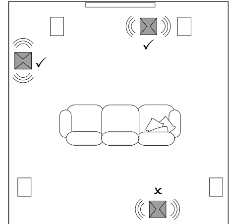
Şekil 1b DB1D, DB2D ve DB3D'nin bir ev sinema (5.1) sisteminde konumlandırılması
