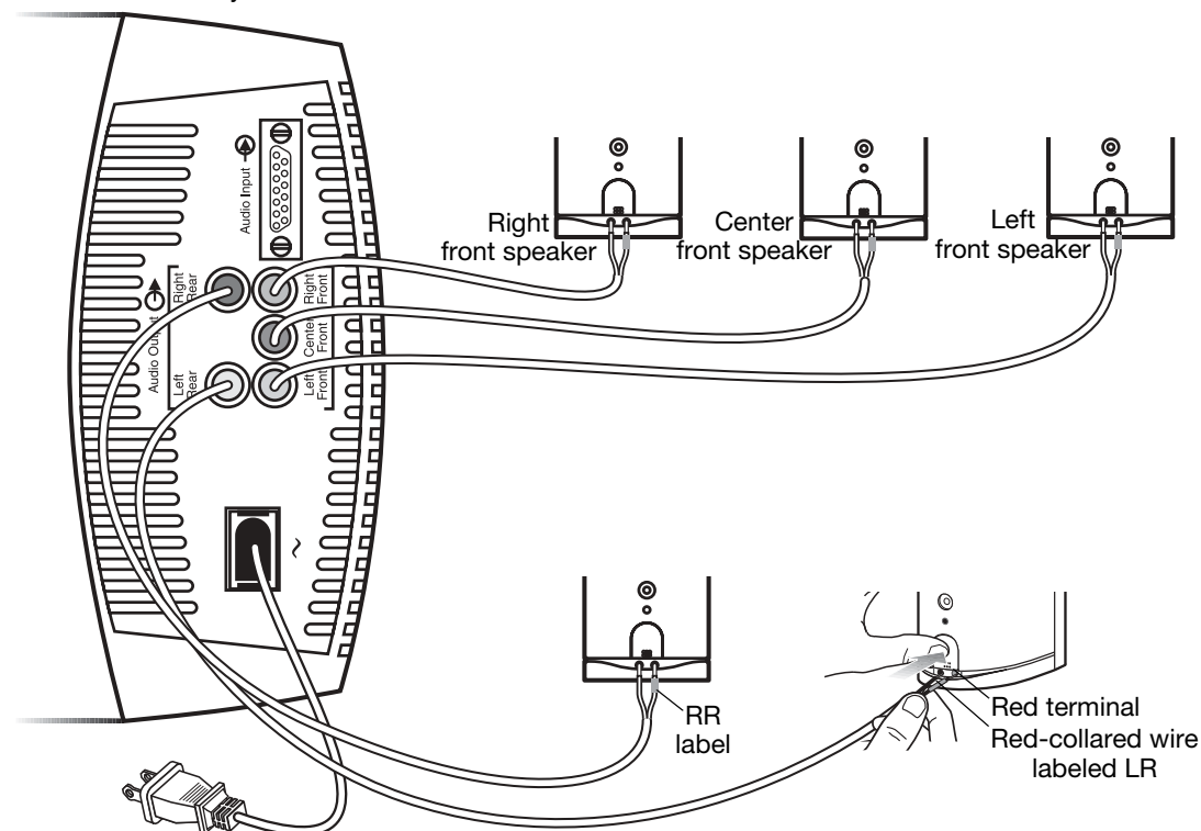
Acoustimass® 10 system module
