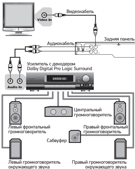
Рис. 4. Подключение к усилителю с декодером Dolby Digital Pro Logic Surround
