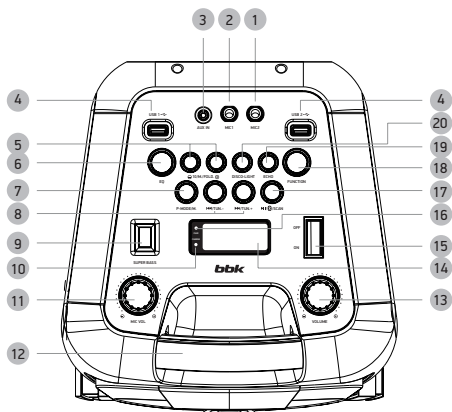
Передняя панель
