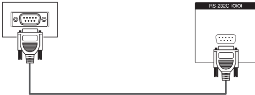
Последовательный управляющий кабель RS-232C (перекрестного типа)
