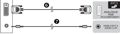
6 Переходной кабель DVI/RGB 7 Стерефонический кабель с минигнездом Ø 3,5 мм
