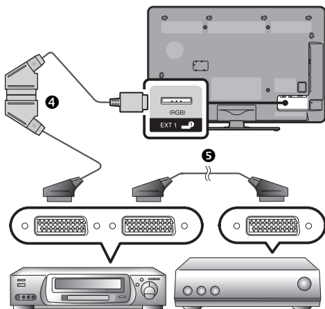
Видеомагнитофон
