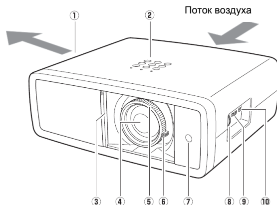
Вид спереди
