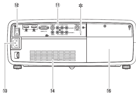
Вид сзади
