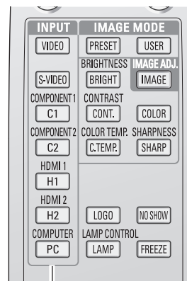
Кнопки INPUT
