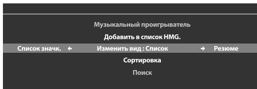
Экран списка
