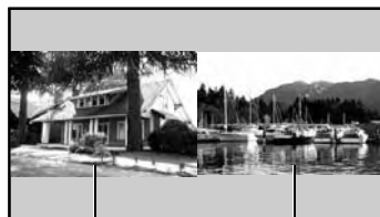
Основной экран
