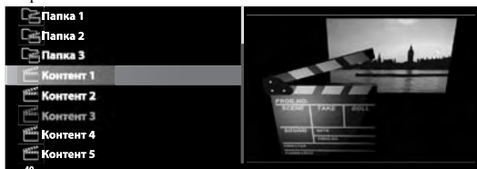
Экран списка
