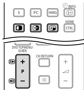
Вспомогательный экран
