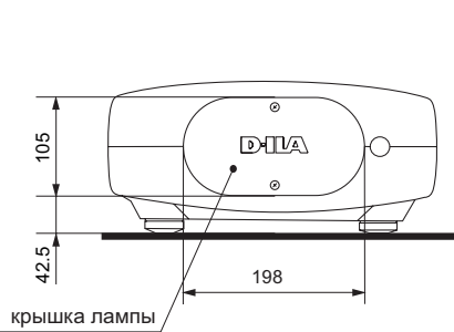
■ Вид сзади
