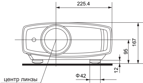
■ Фронтальная
