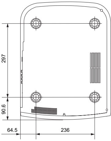
■ Вид снизу
