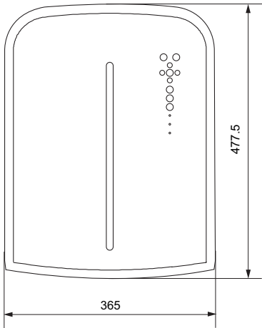
■ Вид сверху
