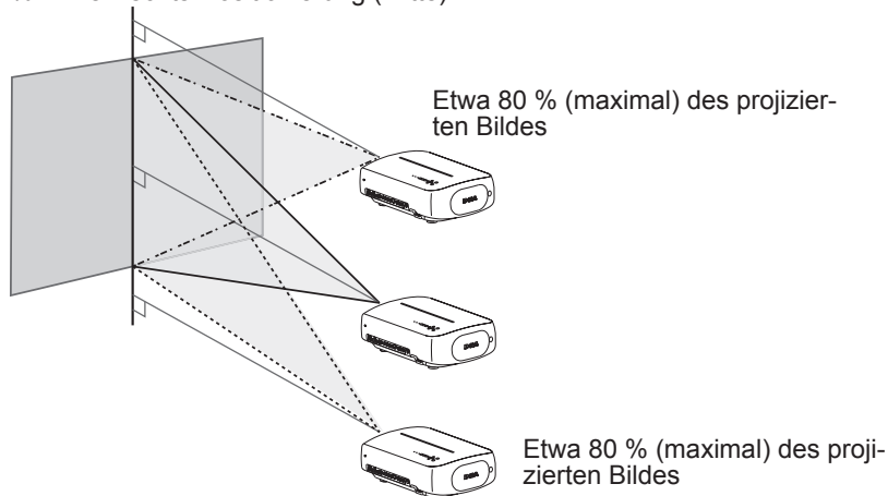
Objektivverschiebungs-Korrelationsschaubild
