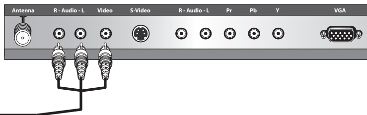
Телевизор
