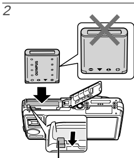
Ручка фиксатора аккумулятора
