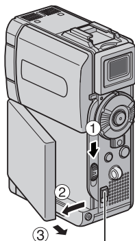
Переключатель BATT.RELEASE
